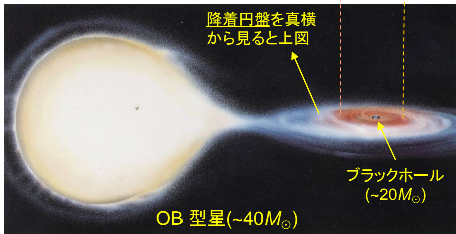
Cyg X-1 の模式図。連星周期:5.6日。 40M ⊙ = 太陽質量の40倍
