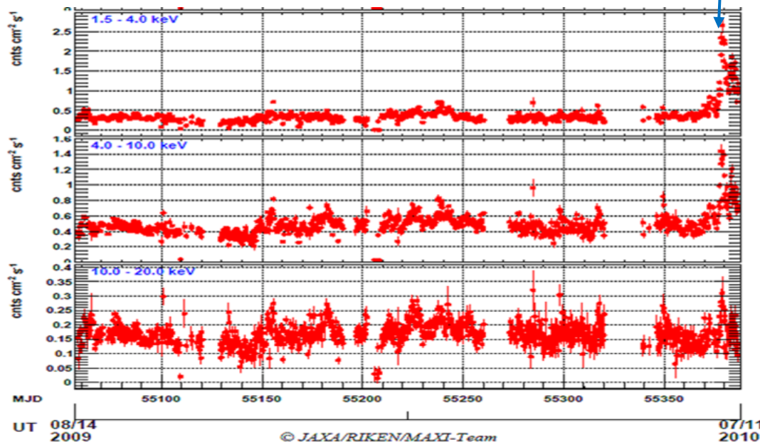
Cyg X-1 のX線3バンドの強度曲線 http://maxi.riken.jp/ ATel 速報Jul. 1
