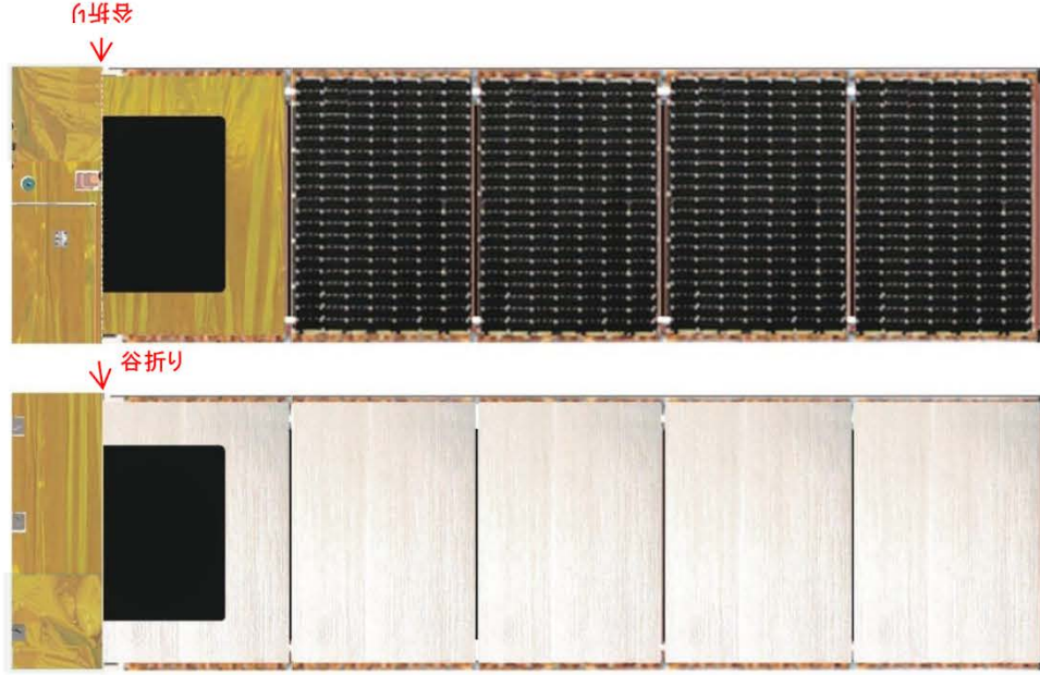
⑫ 太陽電池パドル右翼
